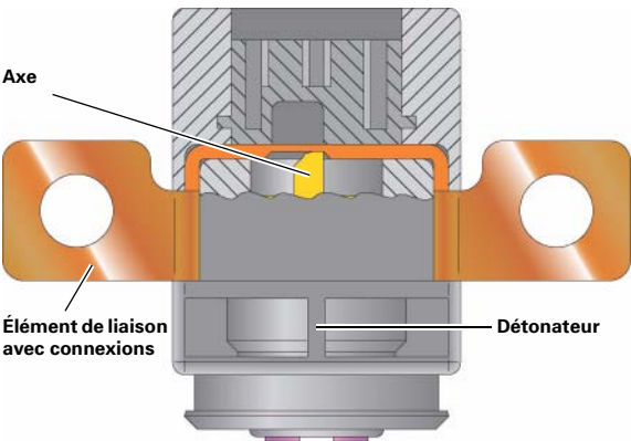
Détonateur de coupure de la batterie
