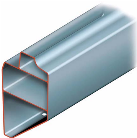
Profilé de seuil Audi A8 Profilé extrudé à trois chambres
