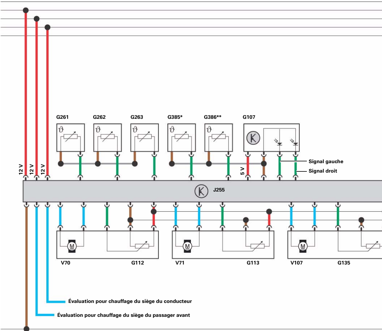
Schéma fonctionnel du climatiseur automatique de l'Audi TT Coupé 07
