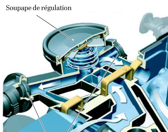
Soupape d'arrêt
