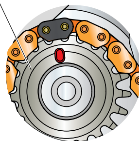
Tendeur hydraulique
