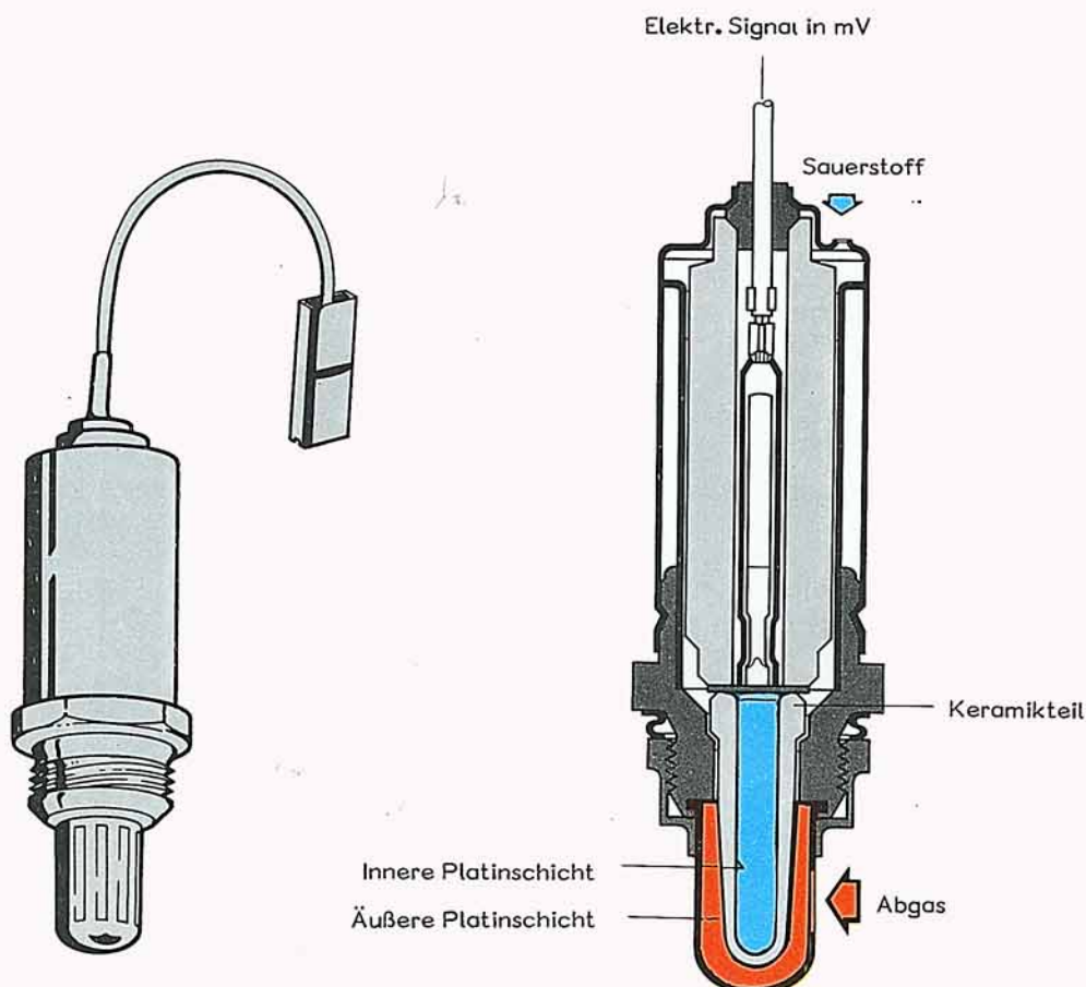
Lambda-Sonde
