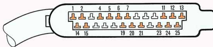
KONTAKTIERUNG DES ZENTRALSTECKERS
