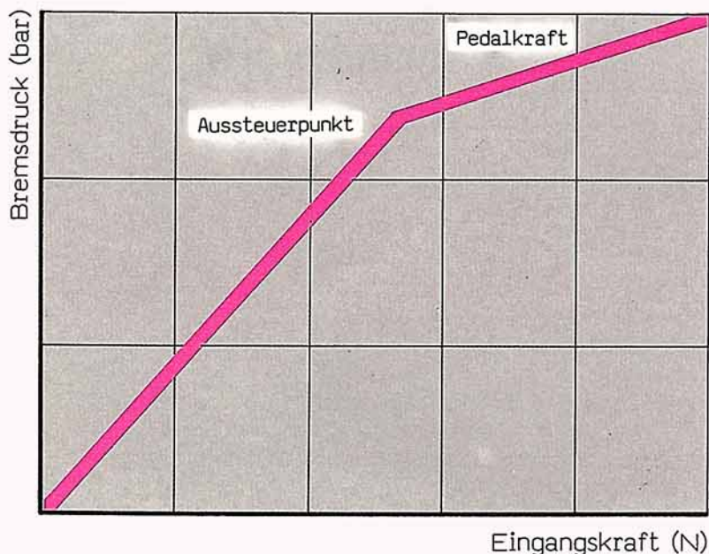
Verstärker-Kennlinie
