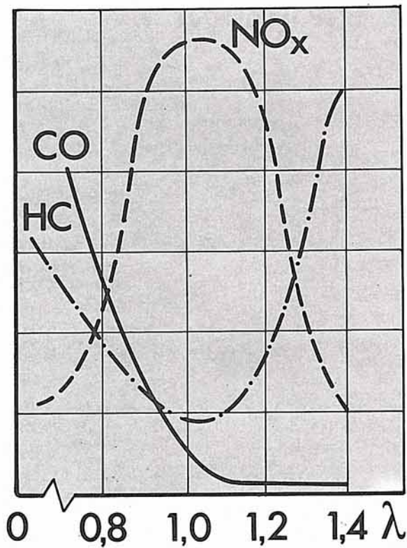
Schadstoffkennlinien beim Ottomotor
