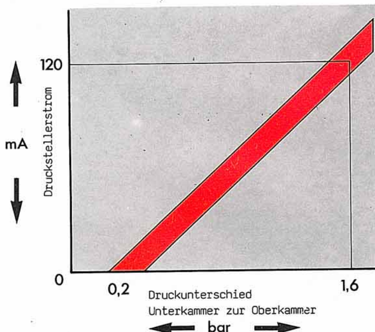
Diagramm-Drucksteller
