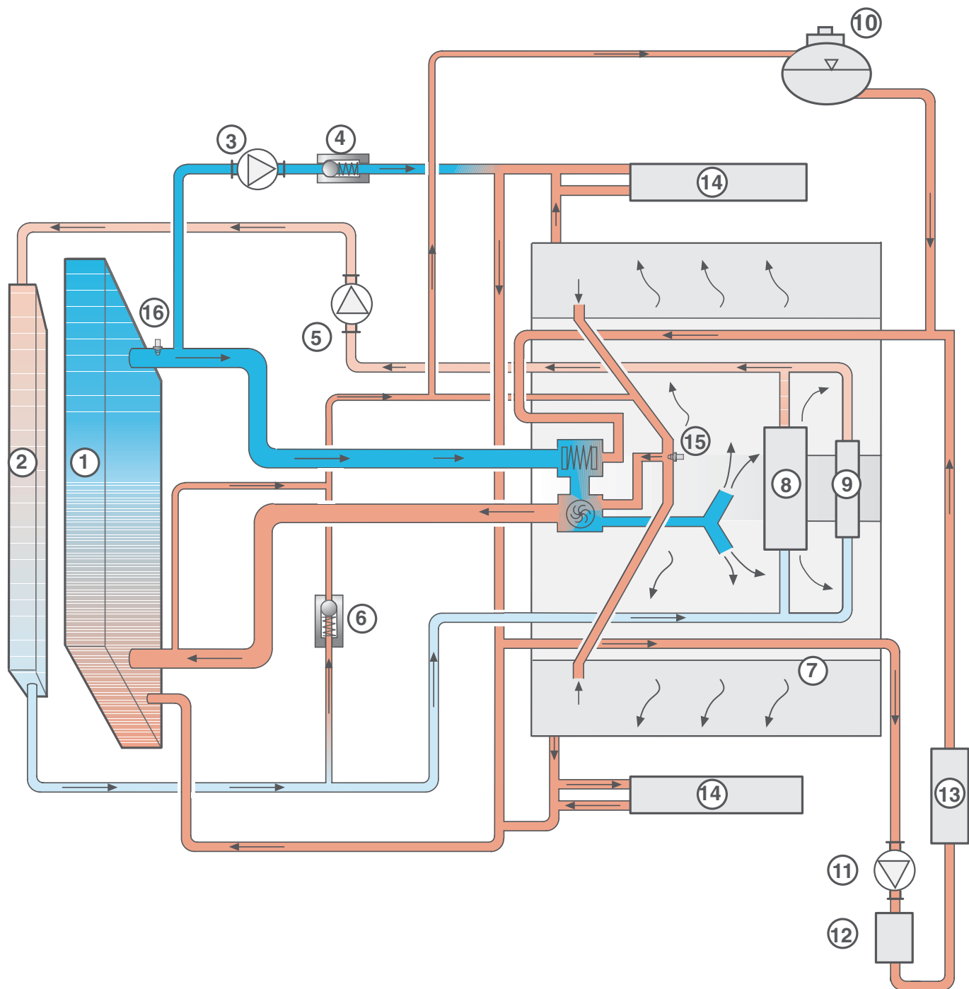
Circuit du liquide de refroidissement
