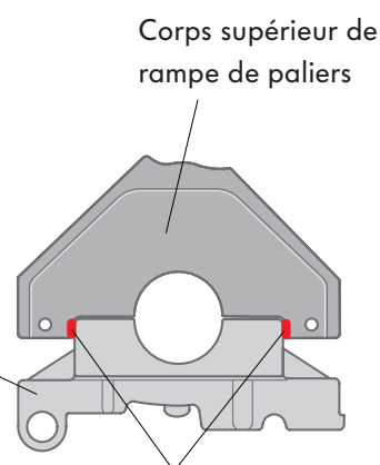
Ajustement sans jeu
