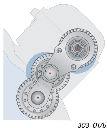
Position à „moteur chaud“
