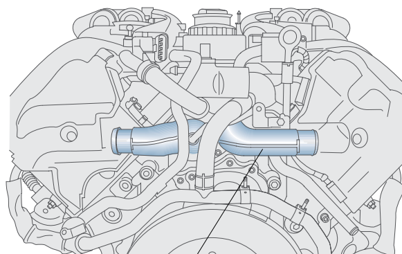
Ajutage de raccordement du boîtier de régulateur du liquide de refroidissement
