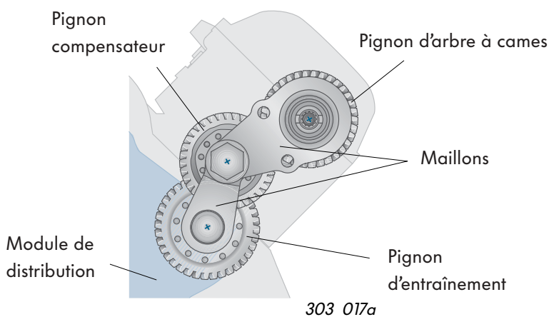
Position à „moteur froid“
