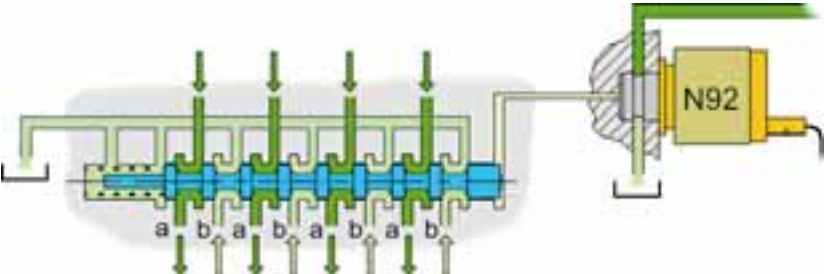
Électrovanne N92 non alimentée en courant
