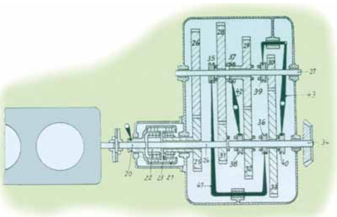
Plan tiré du brevet de Rudolf Franke, datant de 1940
