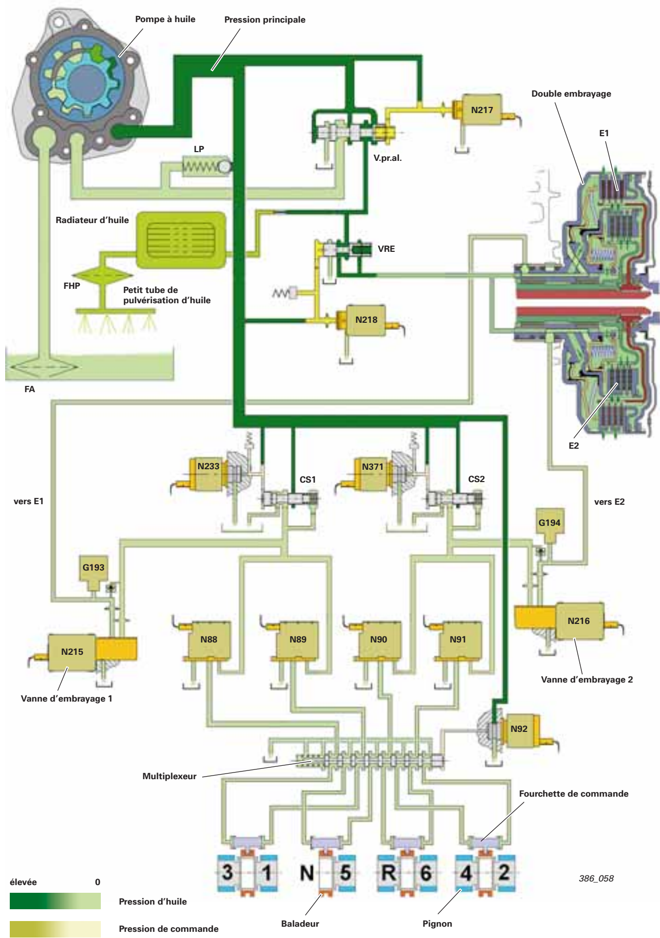
Schéma hydraulique de la boîte 02E
