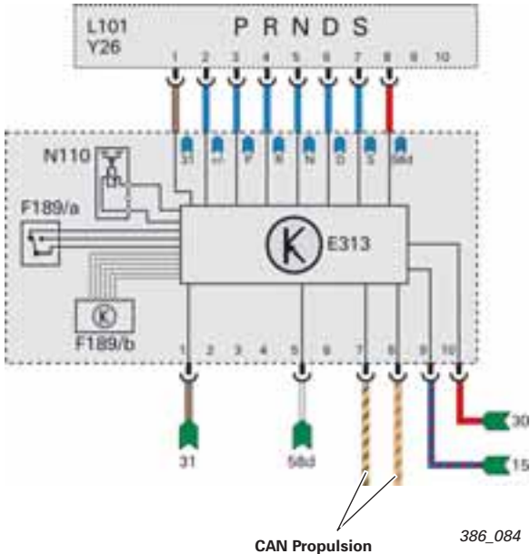
Schéma fonctionnel de la commande des vitesses, Audi TT (8N)
